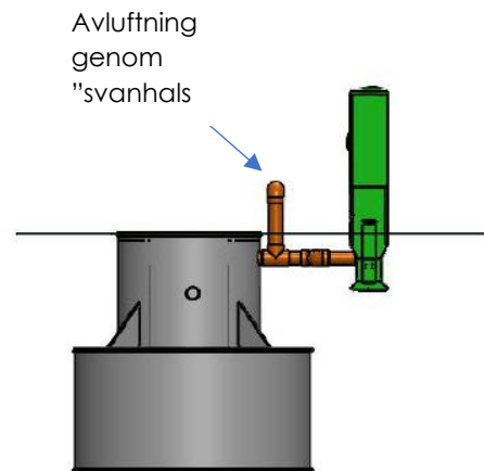
Bilden visar avluftsledningsrörets "svanhals" på anslutningsröret mellan reningsverket och styrskåpet
